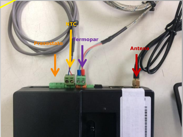
Detalle conexiones
