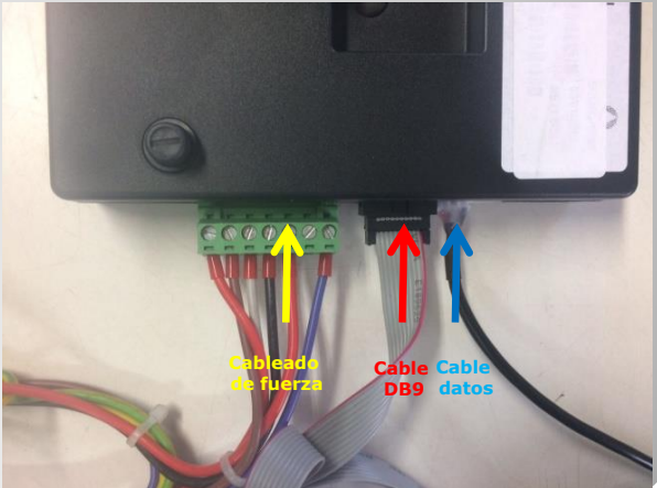
Detalle conexiones
